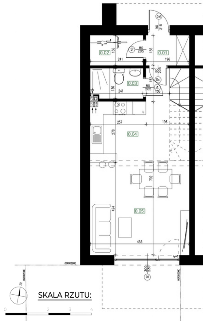
RZUT PARTERU I
