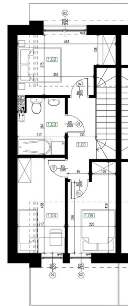
RZUT PIĘTRA I
